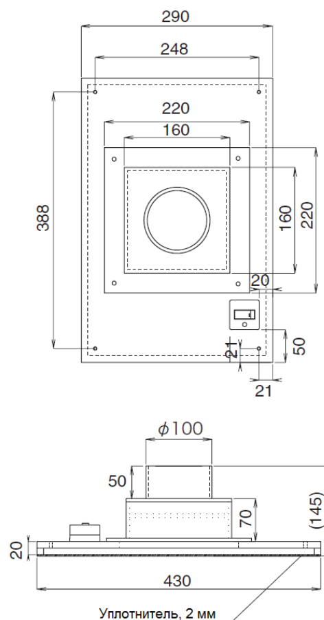
Вентиляционный блок «Тип 1»
