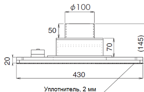
Вентиляционный блок «Тип 1»
