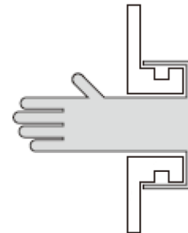
Схема установки перчатки на порт
