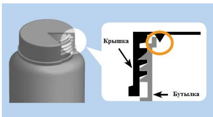
Конструкция крышки бутылок из PE и PP
